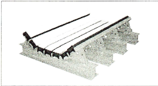
Figure 3 Impact absorbing belt support cradle slika 3 Potpora sa gumenim segmentima za prihvaćanje udara
