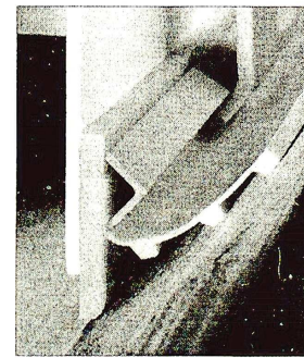
Figure 5 Multiple-layer sealing system slika 5 Višeslojni zaptivni sistem
