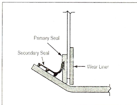
Figure 5 Multiple-layer sealing system slika 5 Višeslojni zaptivni sistem
